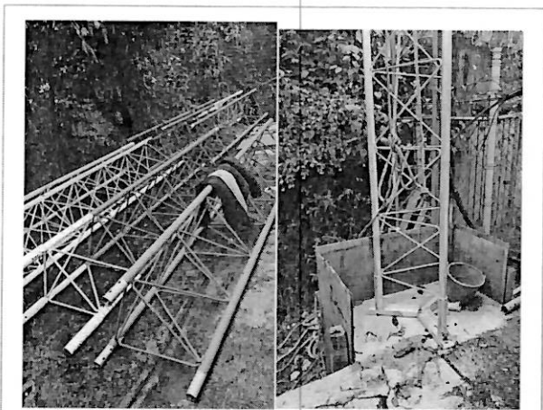
Se suben los tramos de torre, se efectuó el colado de la base de la torre, se instala torre en paralelo con torre de menor carga.
