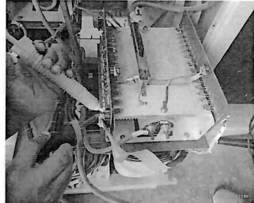
Al hacer una revisión de los tracks se encuentra uno doblado, se sustituyó, también se encuentra un fusible dañado
