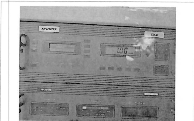
Se puso en operación el transmisor, pero el elemento radiador estaba cerca de la torre que se desmontaría, el transmisor se alarmo con FOOLBACK. Se desmonto el tramo superior que le estorbaba, para quitar la alarma, y al siguiente dia se desmonta la torre vieja.
