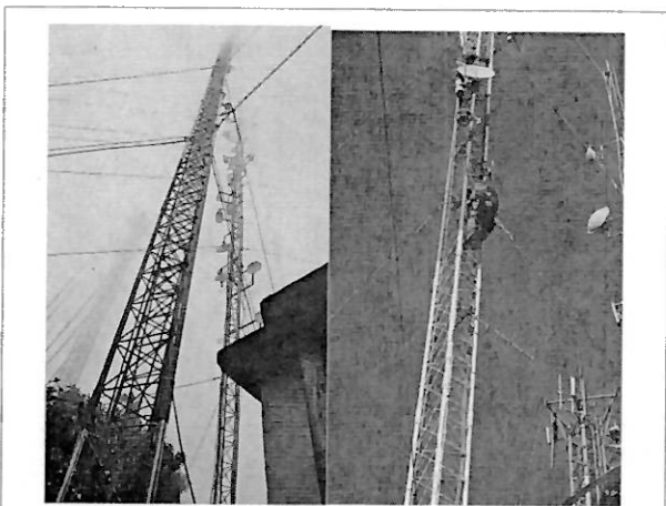
Se levanta torre a la misma altura de la otra, se cambian el elemento radiador, la antena del enlace estudio-planta, cámara y enlace digital.
